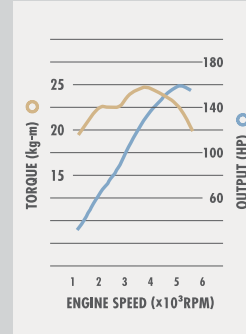
2TR-FE 2.7-litre Gasoline 158HP/5200rpm 24.6kg-m/3800rpm
